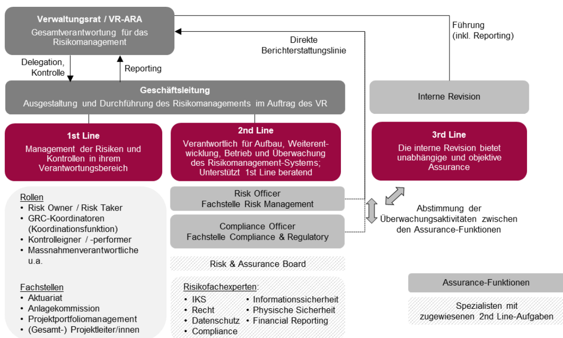
Abbildung 3: Risikomanagementsystem Berichtsperiode
